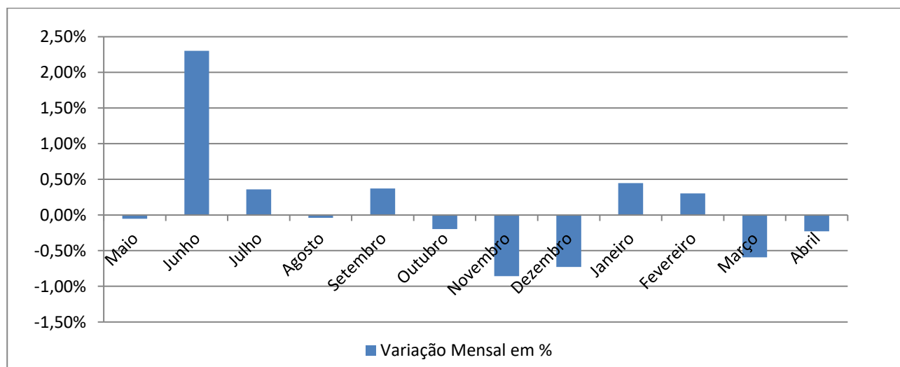
Figura 1 – Variação mensal do Custo da Cesta Básica de Ijuí – Dados em percentuais
